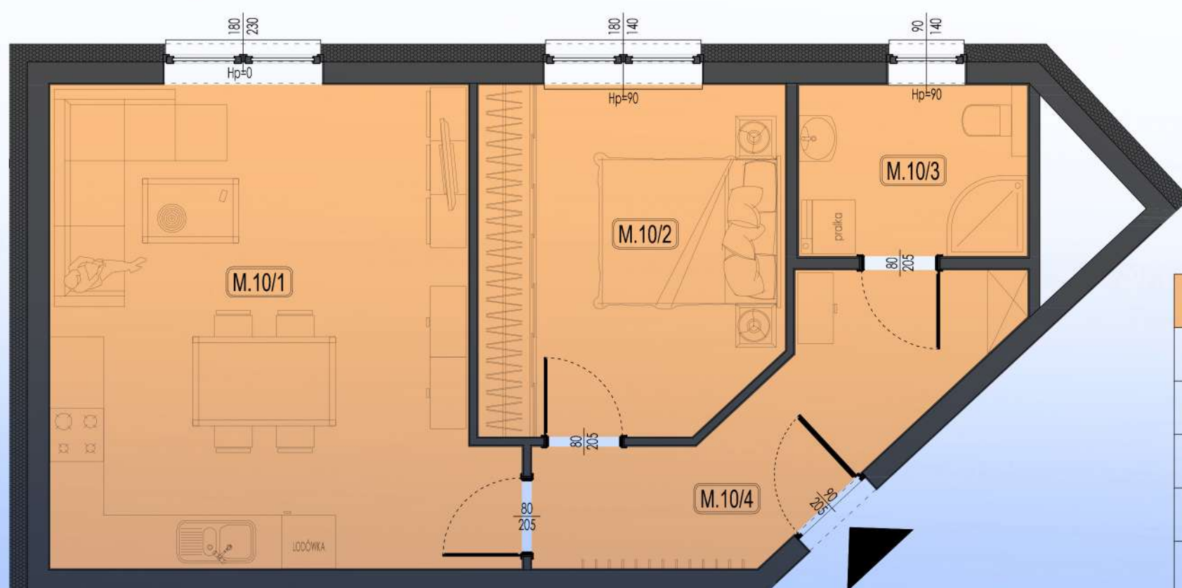
RZUT MIESZKANIA SKALA 1:120
