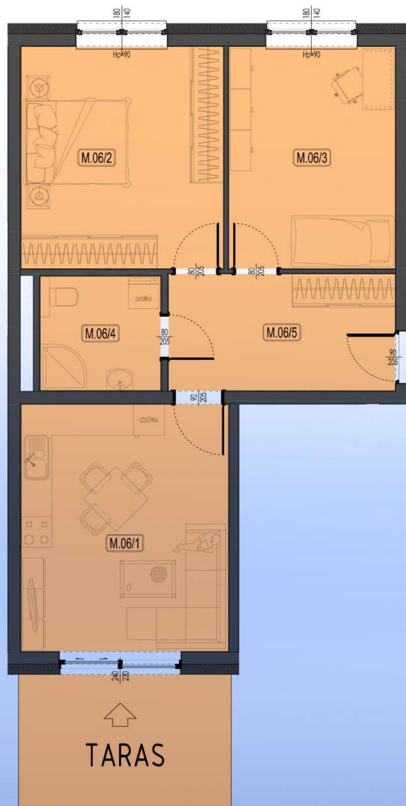
RZUT MIESZKANIA SKALA 1:150
