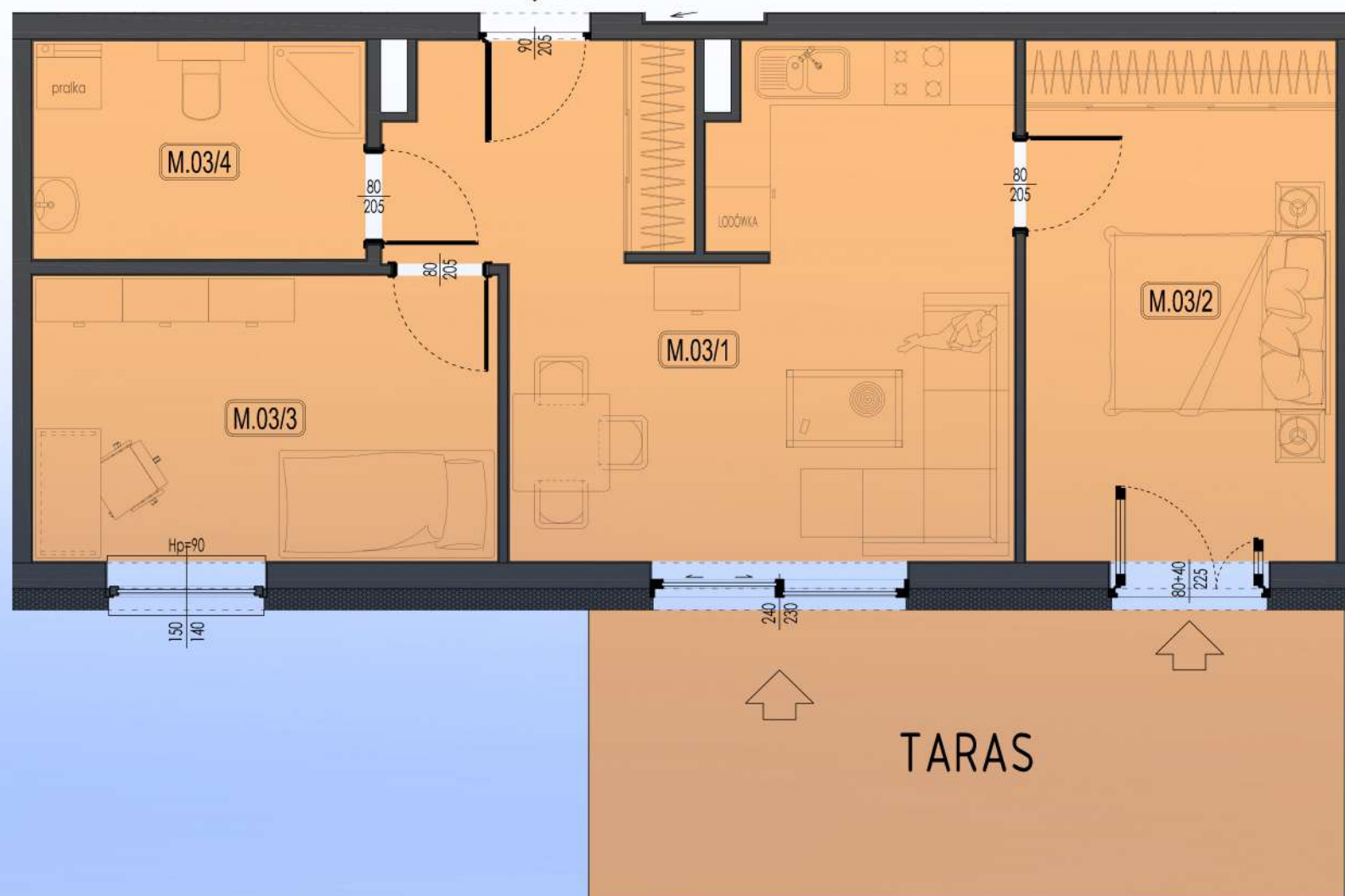
RZUT MIESZKANIA SKALA 1:120
